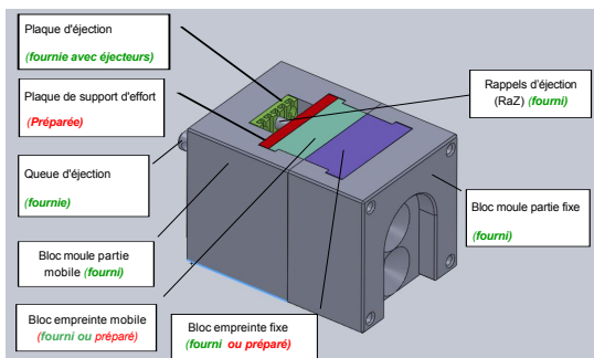
Bloc moule partie fixe
